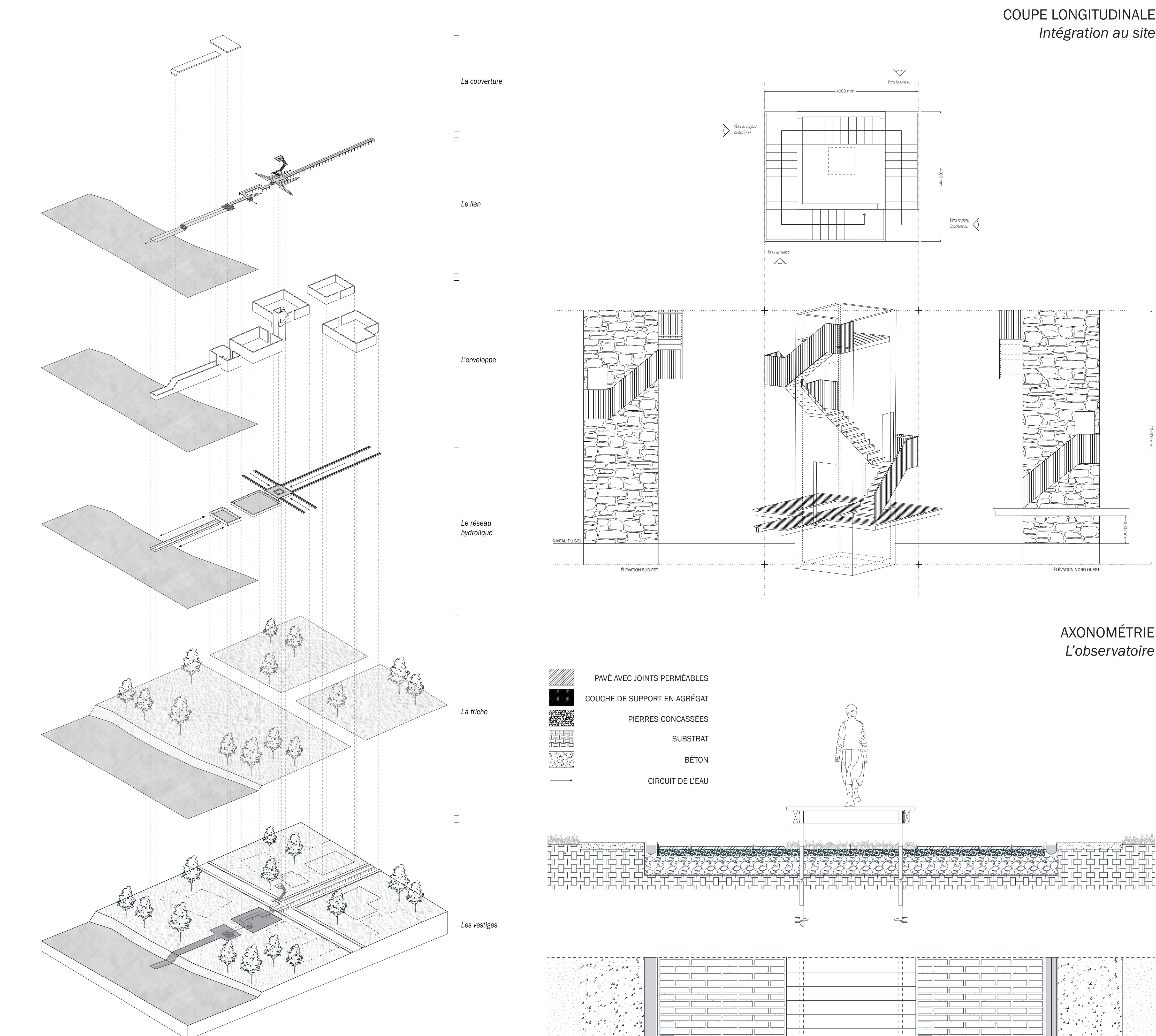
AXONOMÉTRIE ÉCLATÉE Analyse des systèmes et relation avec le site
